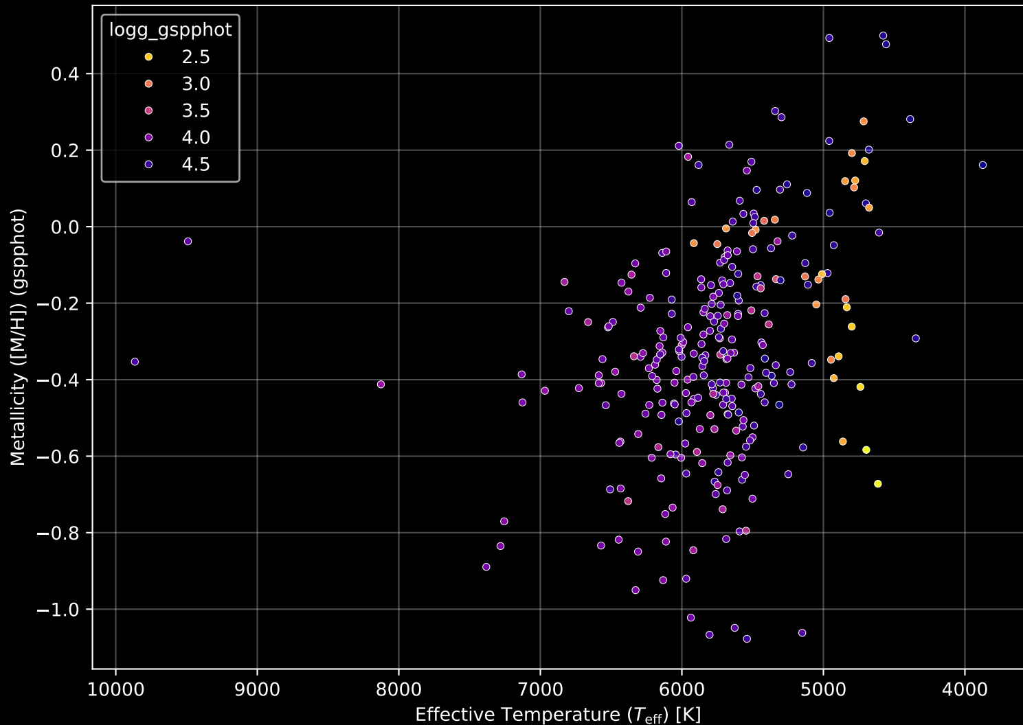
GALAH DR4 Field: [1599] Stellar Population Parameters (n= 286)
