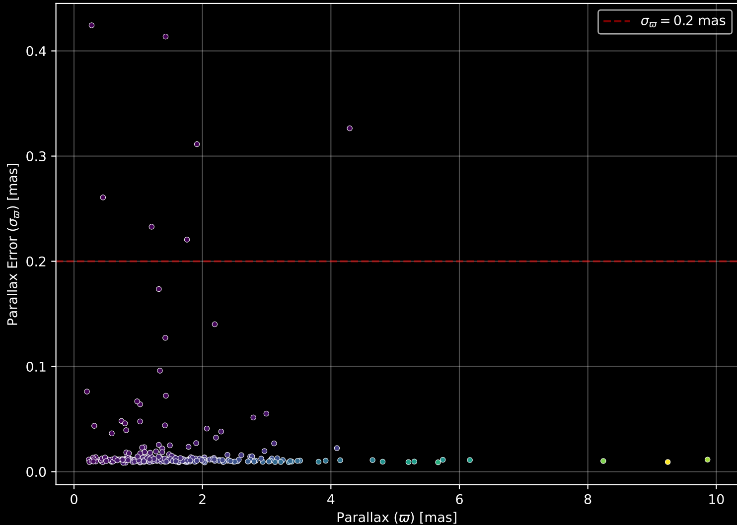
GALAH DR4 Field: [1599] Parallax Quality (n= 286)
