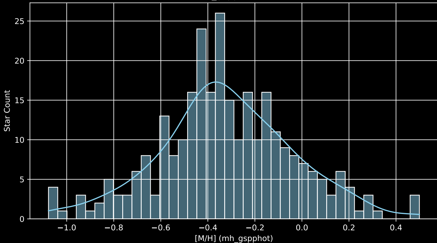
GALAH DR4 Field: [1599] [M/H] (mh_gspphot) (n= 286)
